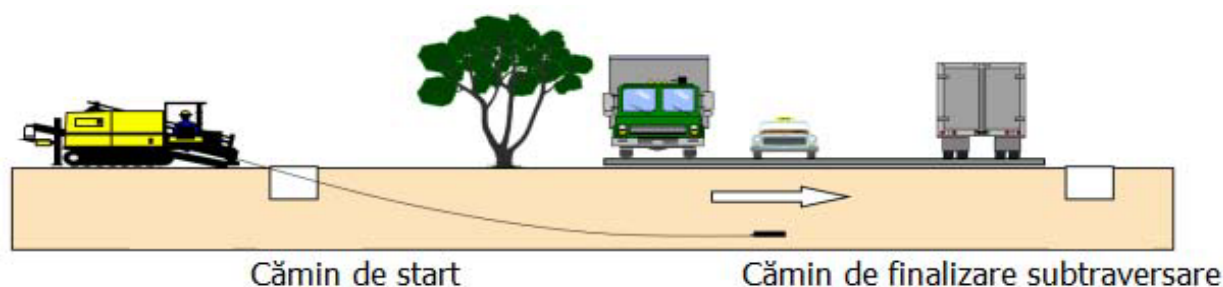
Fig. 2. Foraj dirijat – schema generală
