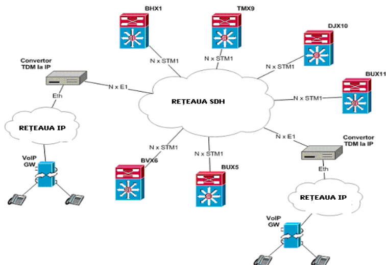
Fig. nr. 4 - Arhitectura rețelei S.C. RCS & RDS S.A.
