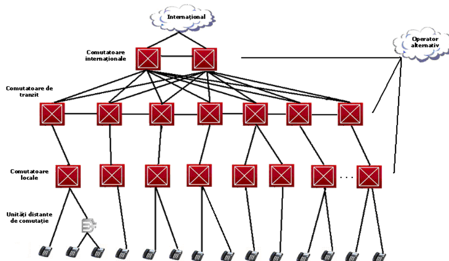
Fig. nr. 3 - Schema generală a rețelei de comutație operate de S.C. Romtelecom S.A.
