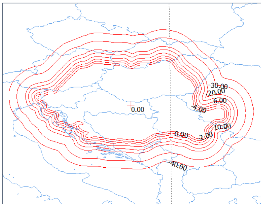
Figura 5.5 – Acoperirea spațială a României din poziția orbitală 26,5° est (ROU-MILSATCOM3-26.5E)
