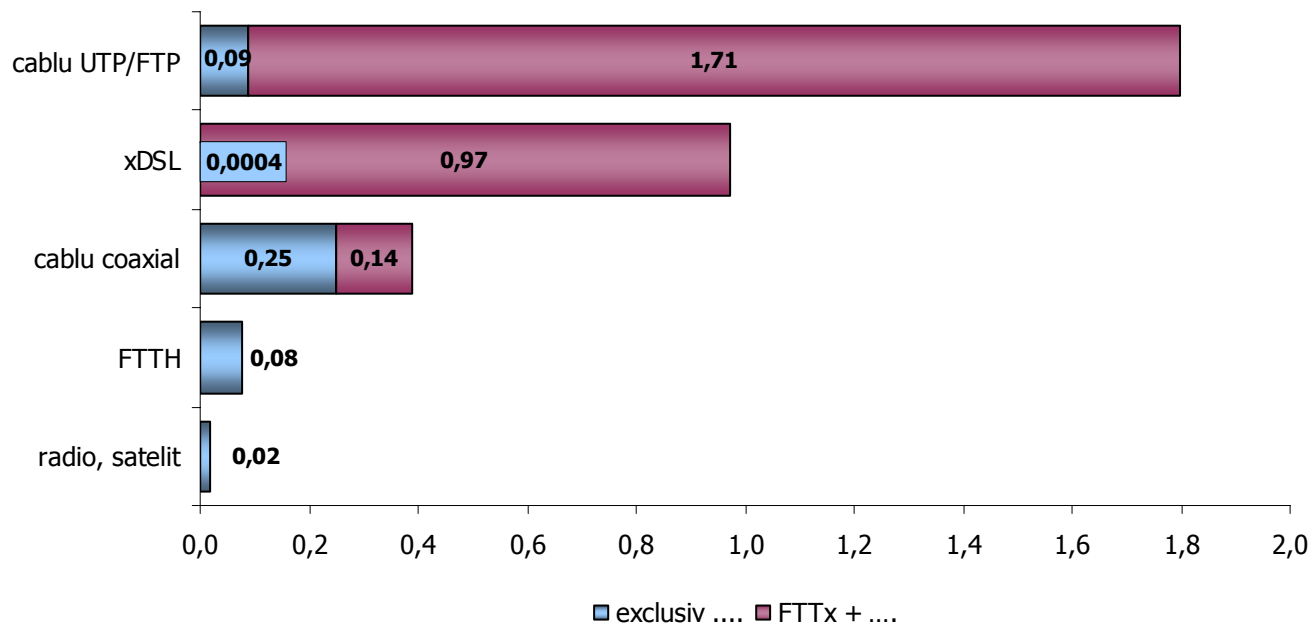
Fig 2.2. Structura conexiunilor de acces la internet în bandă largă la puncte fixe, în funcție de utilizarea tehnologiei FTTx, la 31.12.2011.
