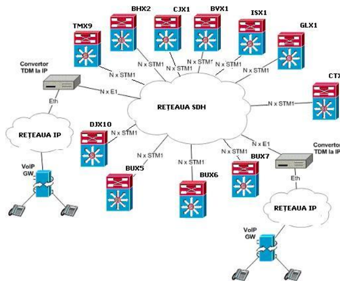
Figura nr. 5.8. – Arhitectura rețelei RCS & RDS S.A.
