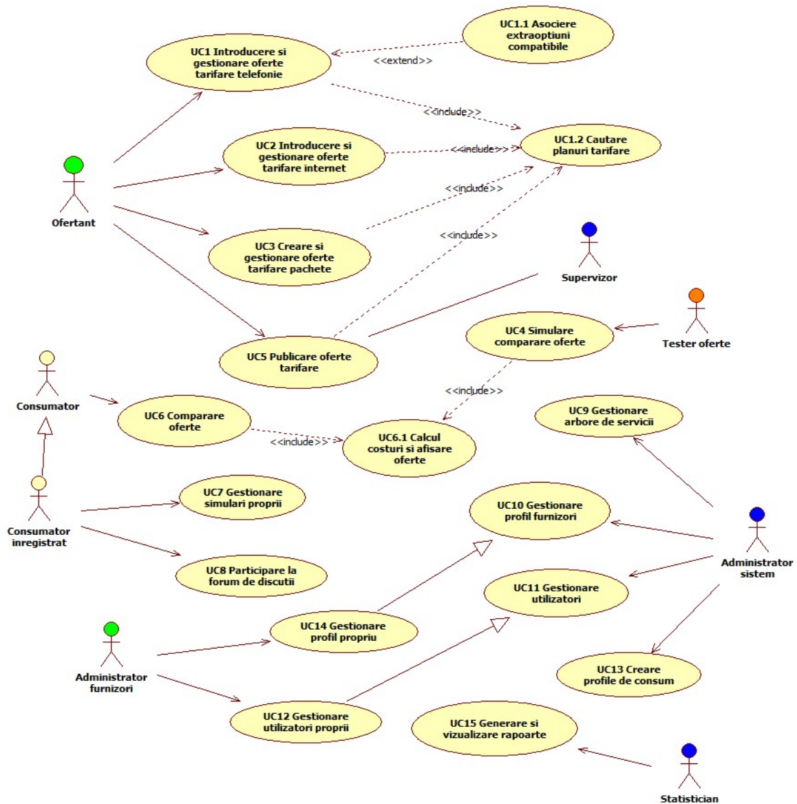
Diagrama cazurilor de utilizare
