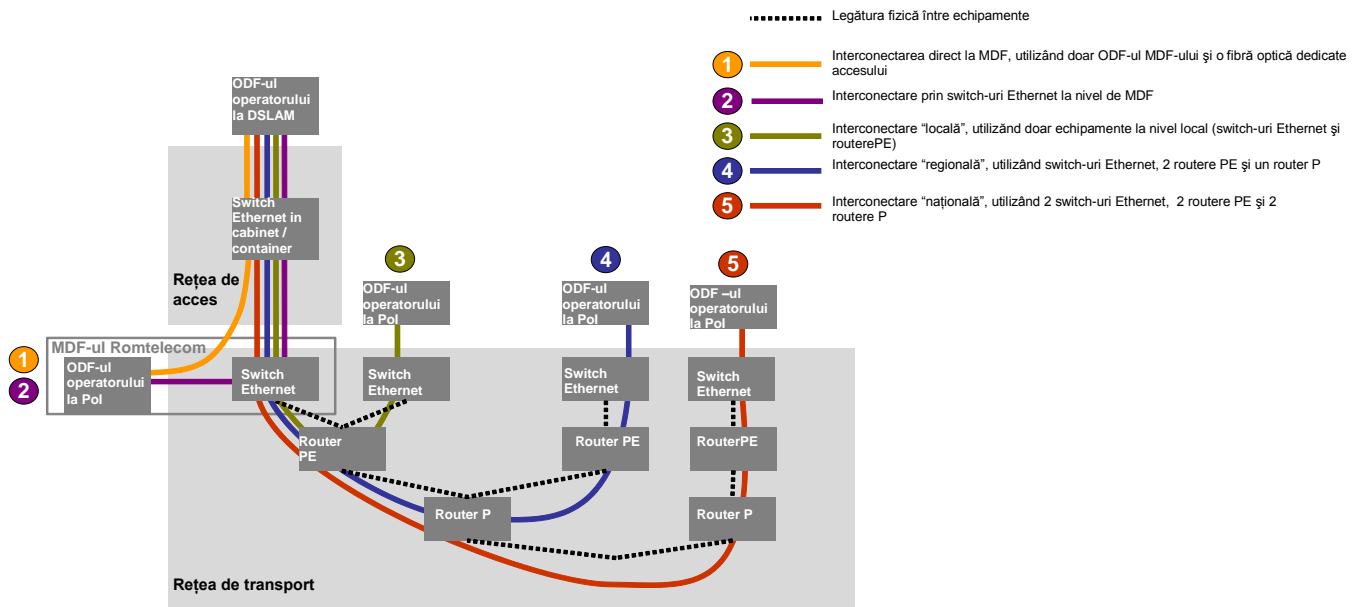
Figura 1. Reprezentarea grafică a serviciilor 1-5 „backhaul” pe suport Ethernet
