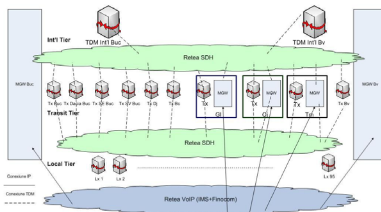
Figura nr. 3.2.2. Schema generală a rețelei de comutație operate de S.C. Romtelecom S.A.
