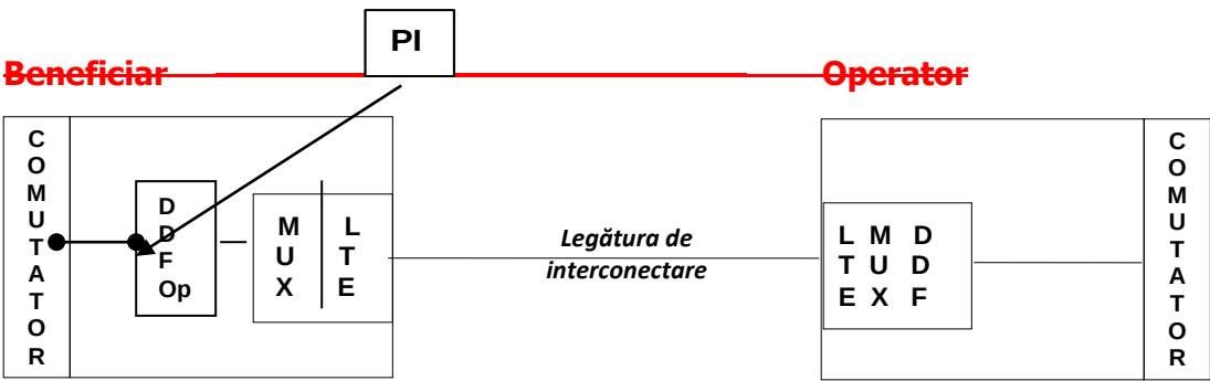
FIGURA 1— INTERCONECTARE DIRECTĂ ÎN SPAȚIUL BENEFICIARULUI (EXEMPLU)
