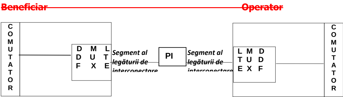
FIGURA 2— INTERCONECTARE DIRECTĂ LA UN PUNCT INTEREDIAR (EXEMPLU)
