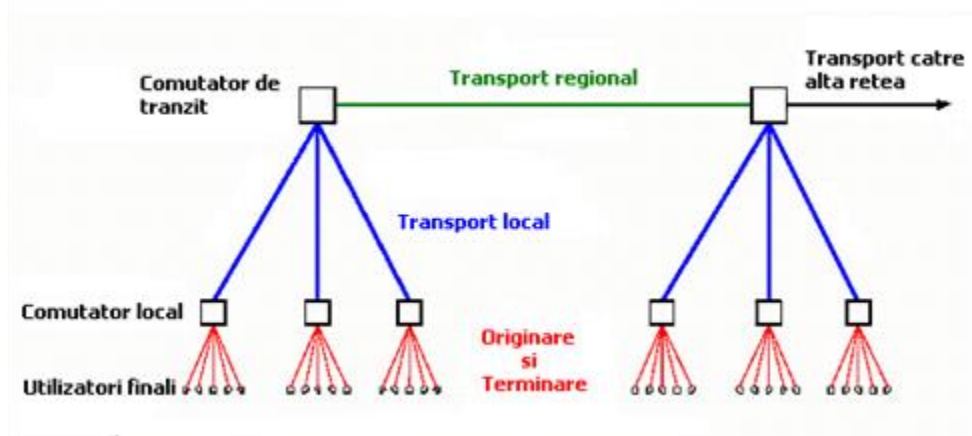
Figura nr. III.2. Prezentare generică a structurii și funcționalității serviciilor de interconectare – origine, terminare și tranzit în cazul unei rețele ierarhice, respectiv în cazul unei rețele IP
