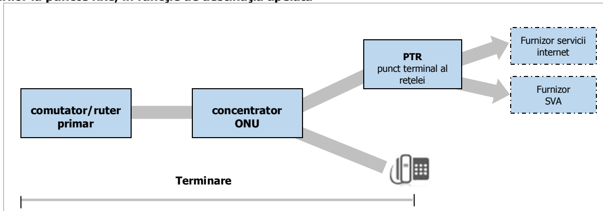
Figura nr. III.6. Schemă generală a segmentului de rețea corespunzător furnizării serviciilor de terminare a apelurilor la puncte fixe, în funcție de destinația apelată
