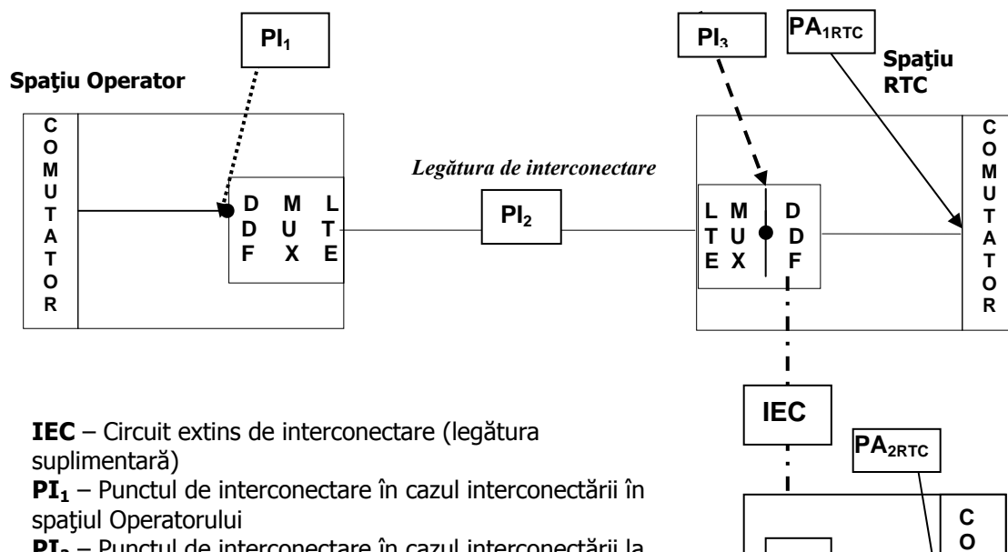
Figura 4 – Interconectare cu circuit extins (exemplu)
