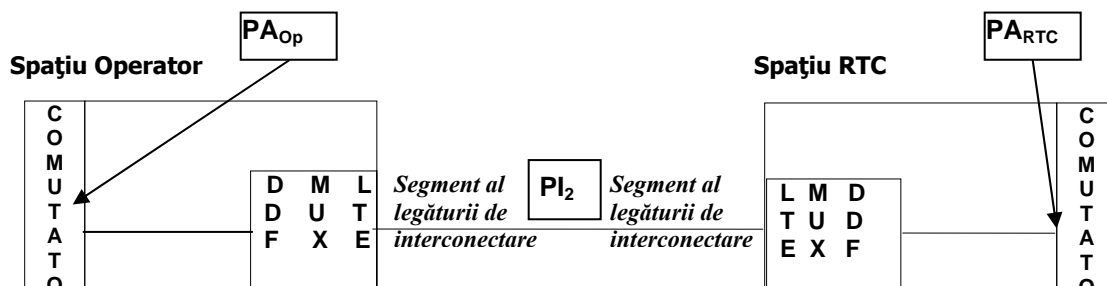
Figura 2 – Interconectare directă la un punct intermediar (exemplu)
