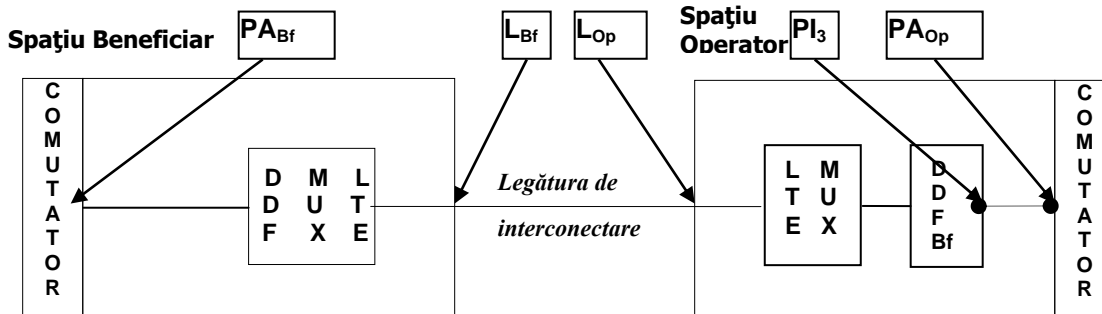
Figura 3 – Interconectare directă în spațiul Operatorului (exemplu)
