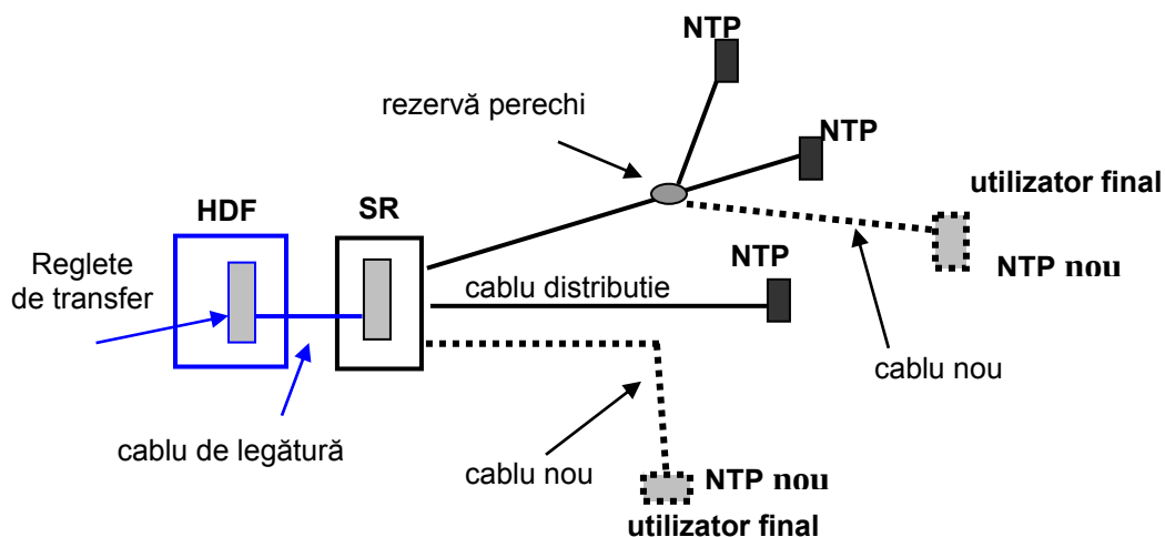
Fig.4 Posibilități de acces la subbucla locală pe o pereche nouă
