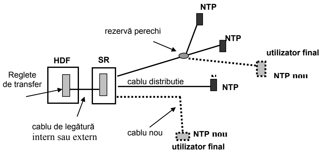
Fig.2 Posibilități de acces la subbucla locală pe o pereche nouă
