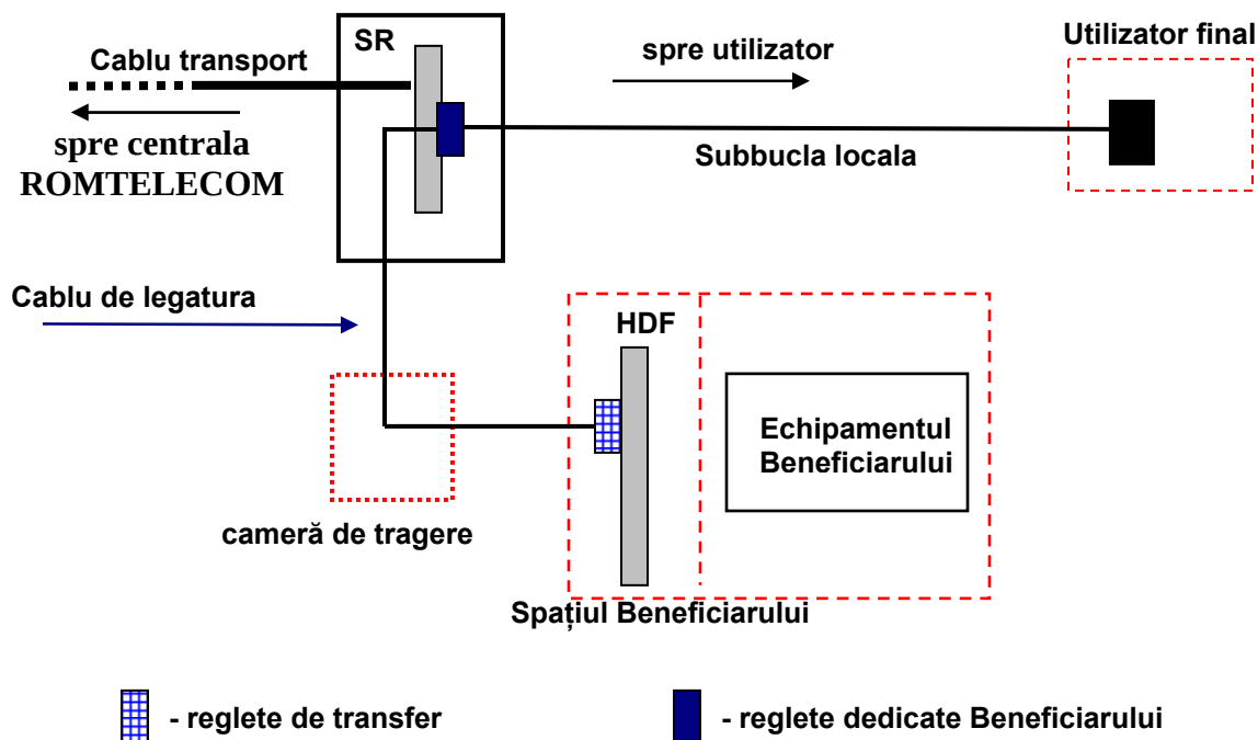
Fig.4. Legătura dintre SR și HDF
